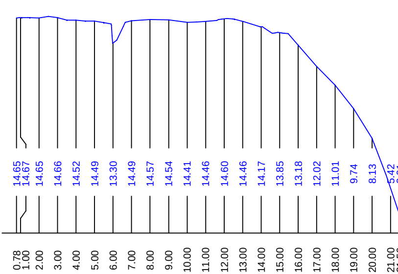
Řez 8
