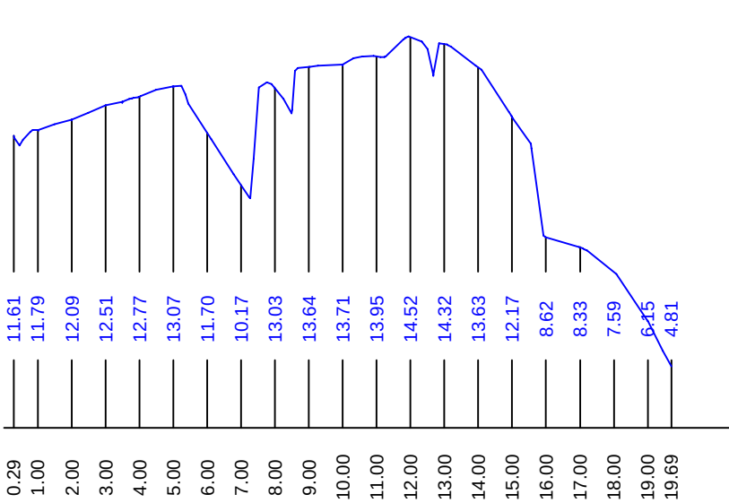
Řez 6
